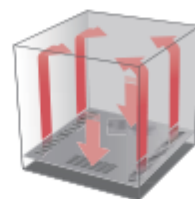
对流模式
